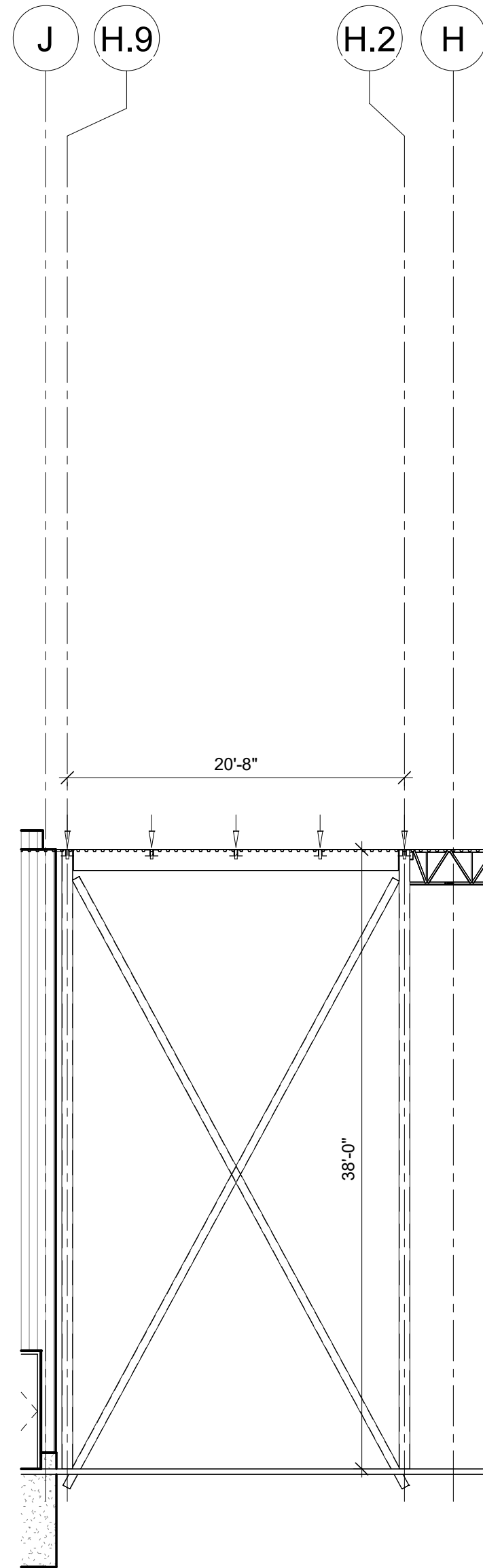
AXE 6 DE H.2@H.9 1/8" = 1'-0"
