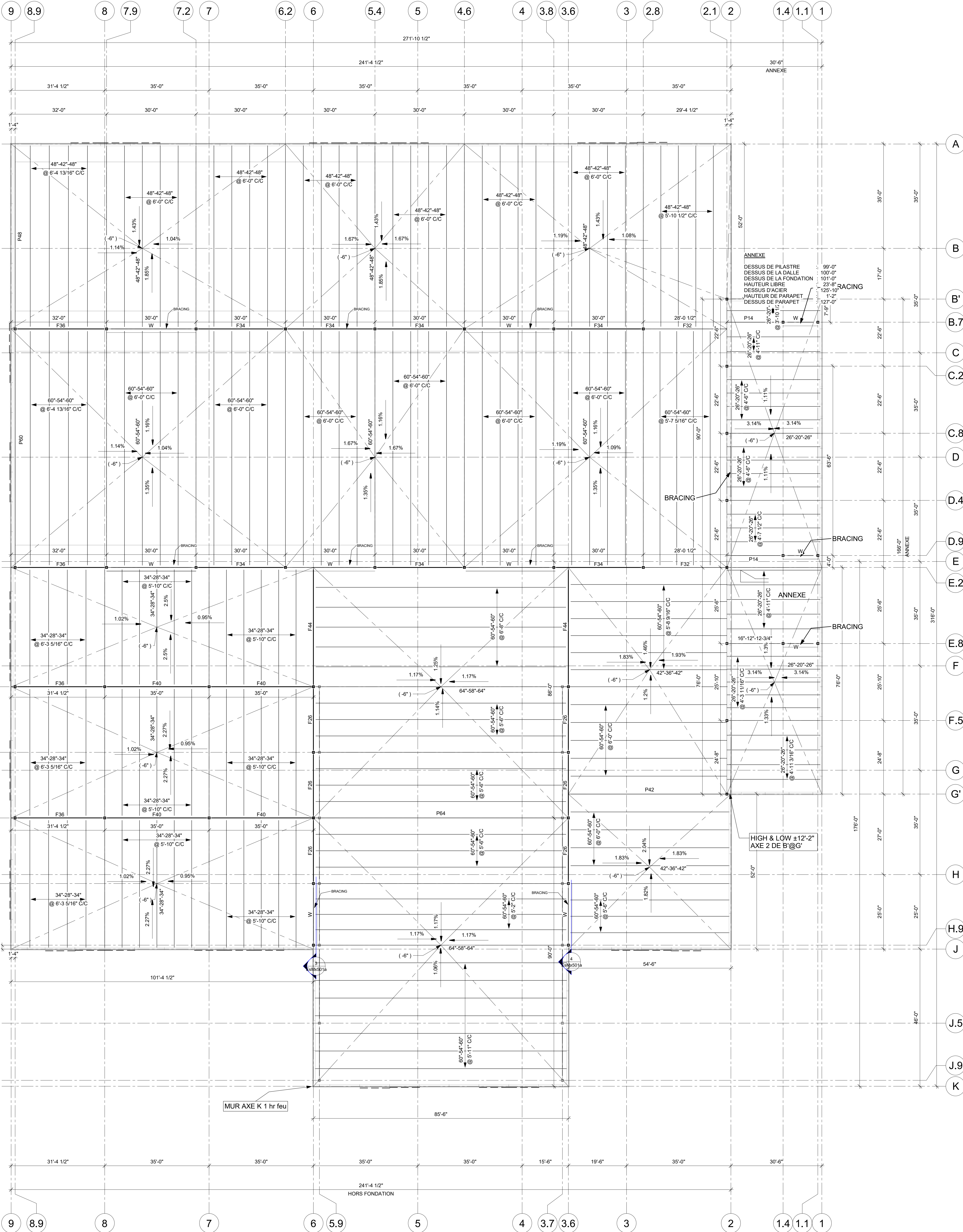
PLAN DE TOIT 1:156
