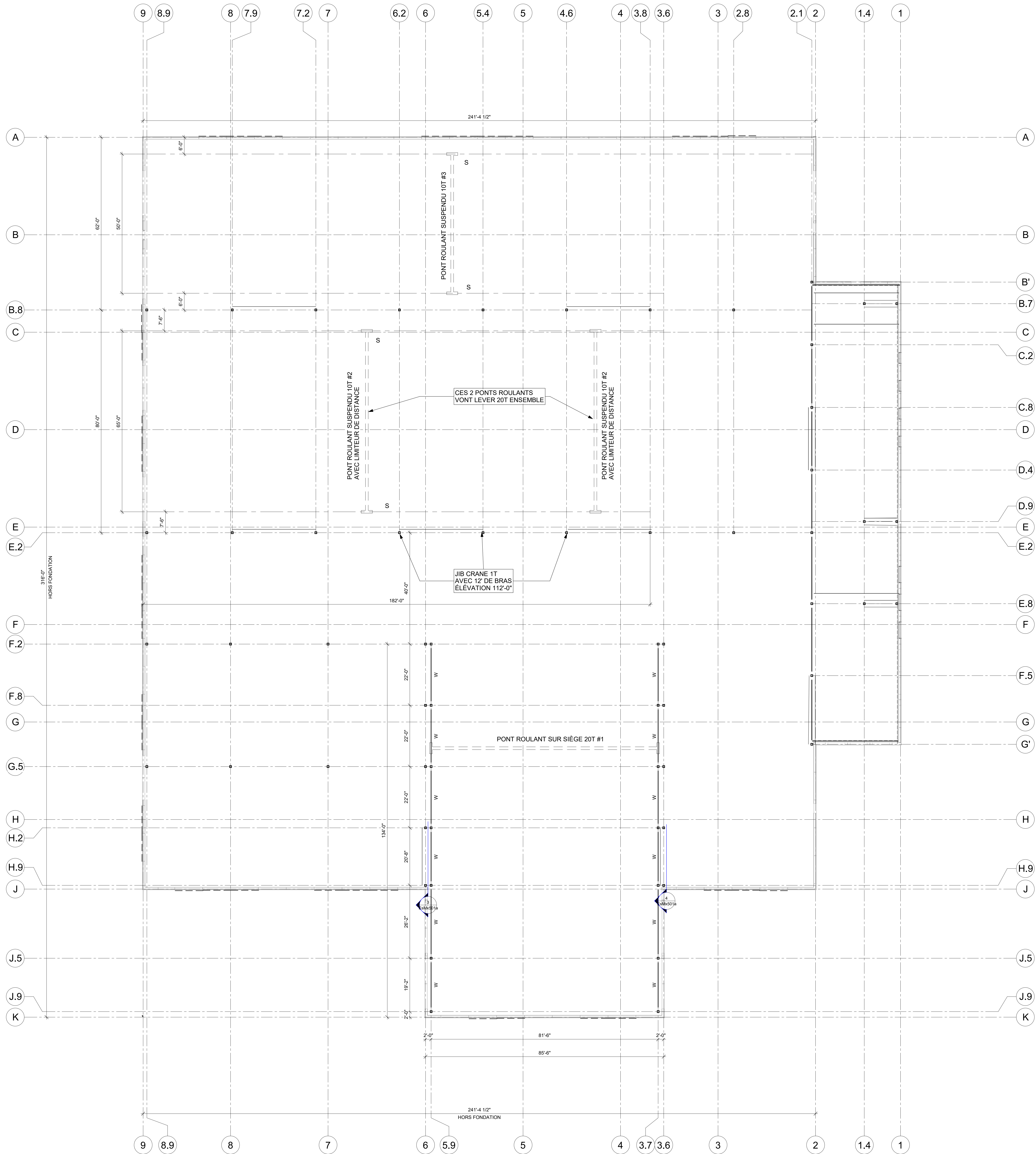
PLAN PONTS ROULANTS 1 : 100
