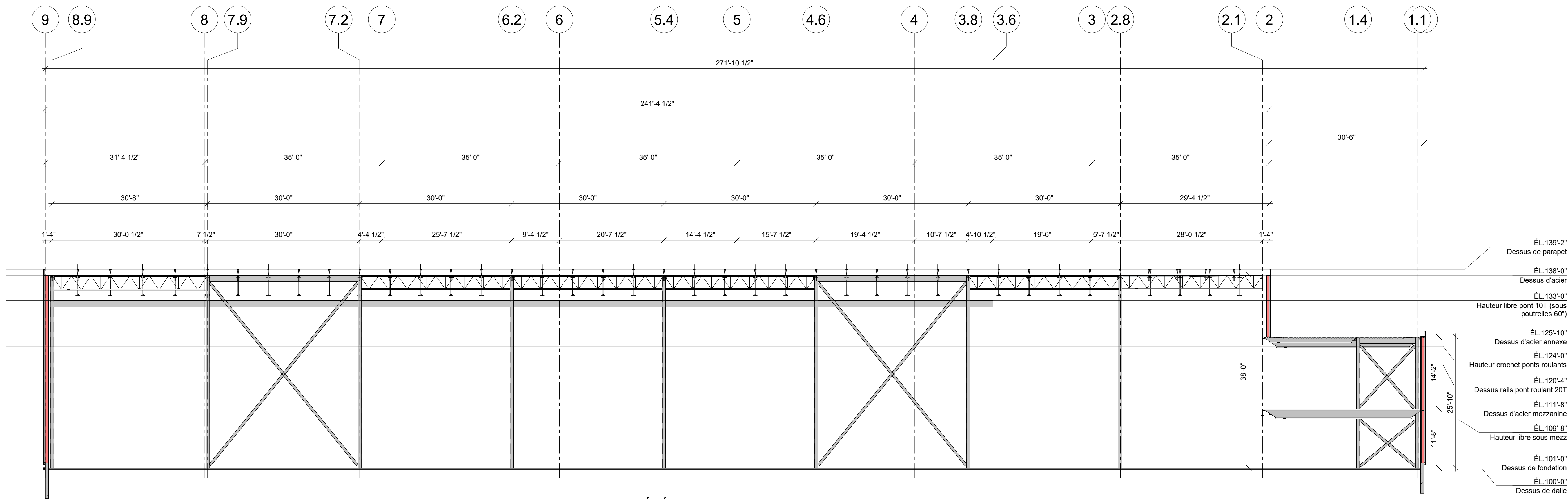
ÉLÉVATION AXE B.8 (STRUCTURE)(SUD) 3/32" = 1'-0"
