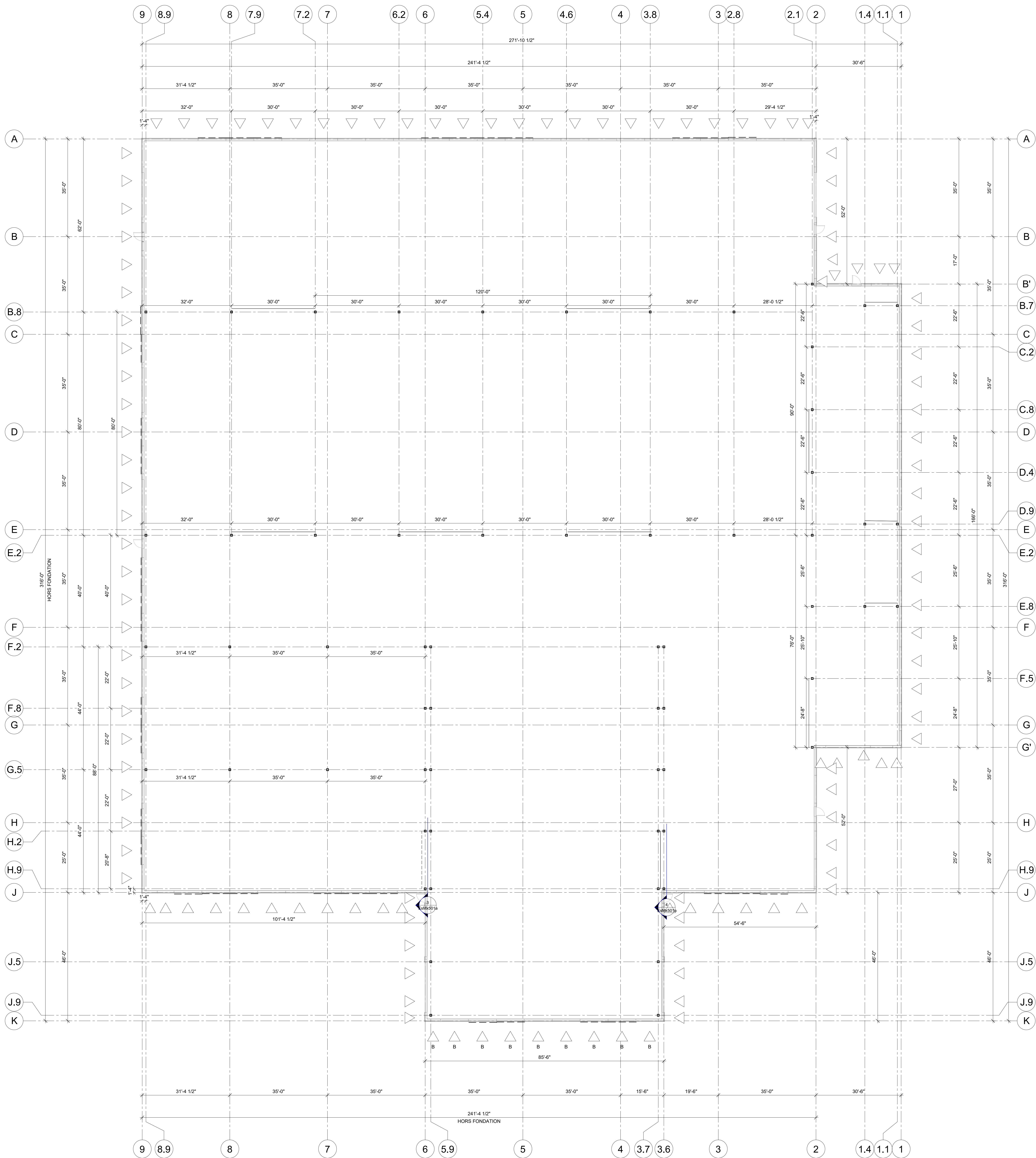
PLAN D'ANCRAGE 1:156
