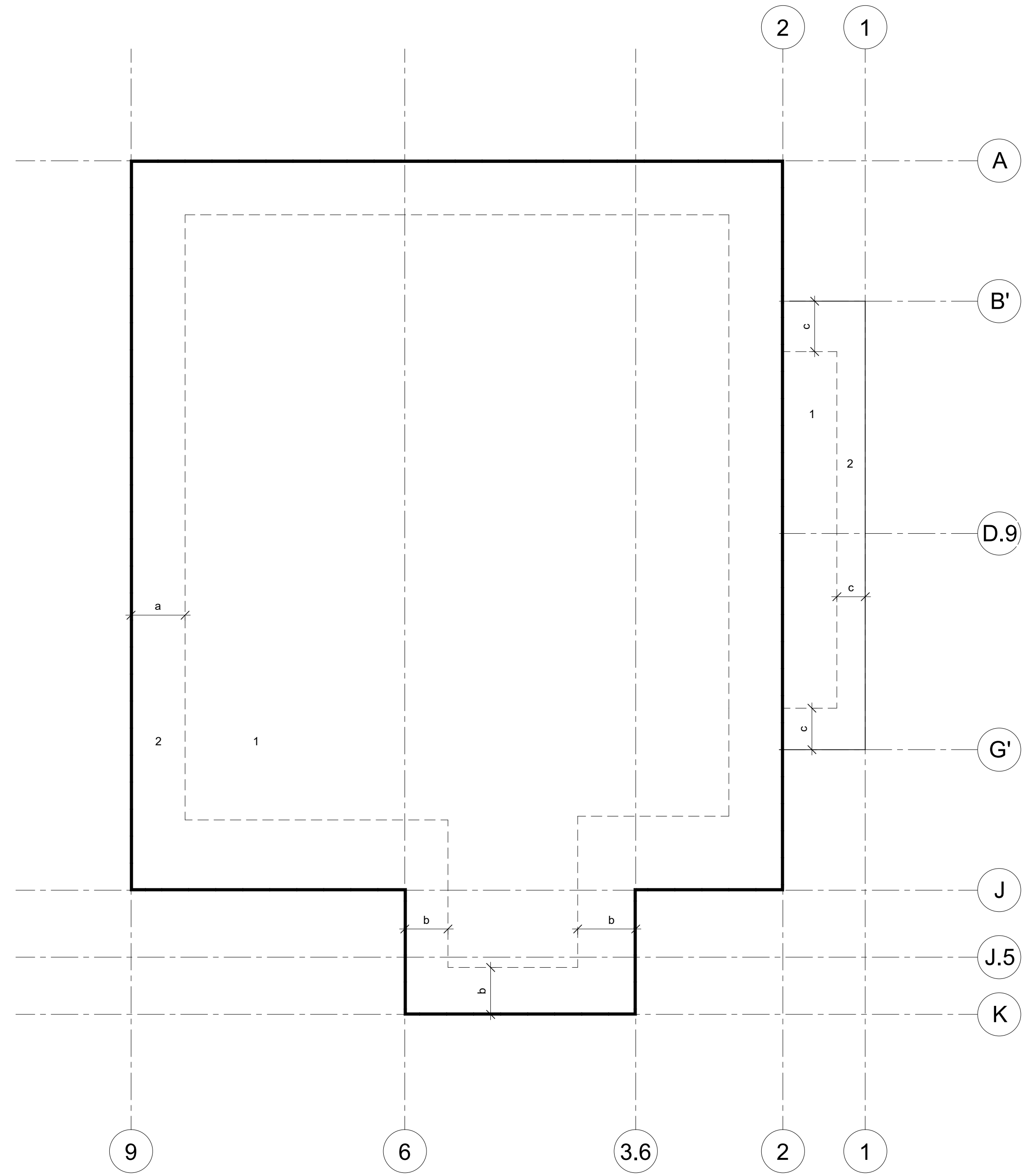
DIAGRAMME DE SOULEVEMENT BRUT (NON PONDERE)
