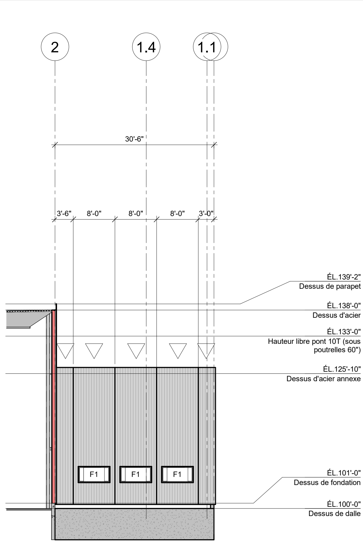
ÉLÉVATION AXE G' (SUD)
