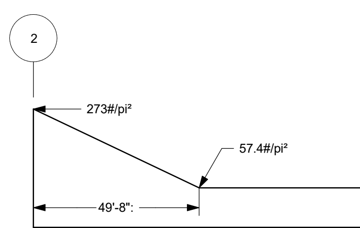
ACCUMULATION DE NEIGE
