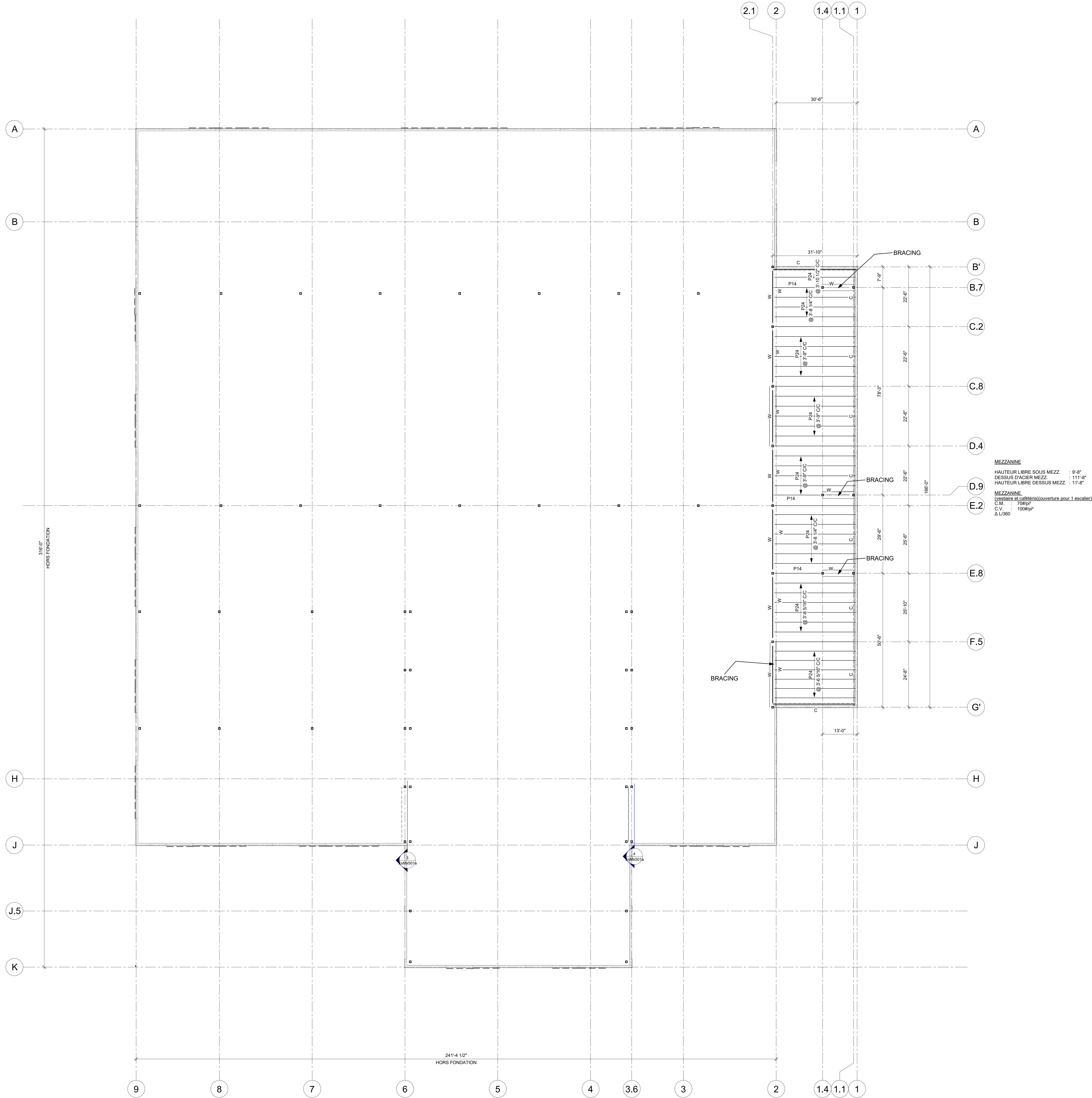
PLAN DE MEZZANINE 1:156
