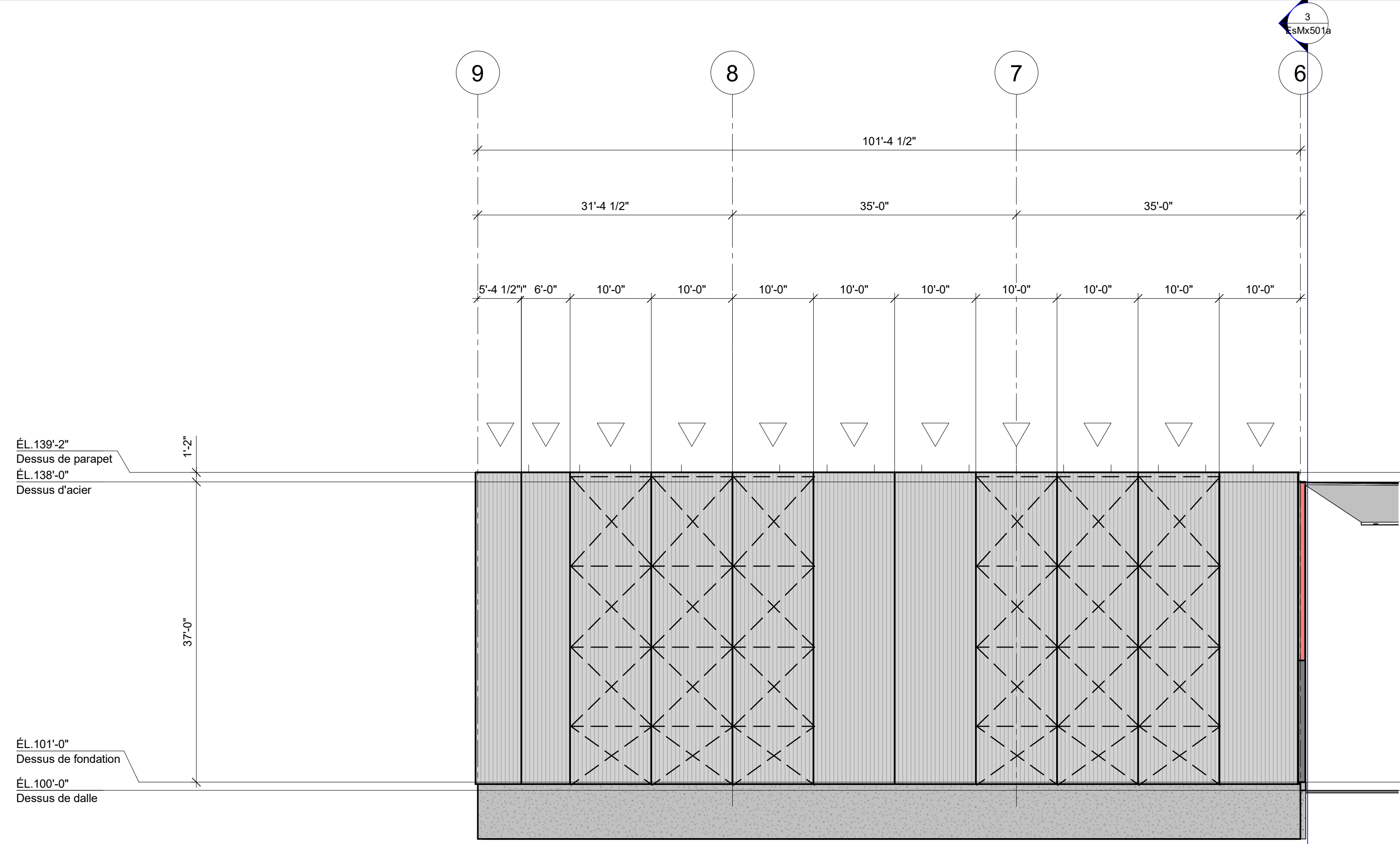
ÉLÉVATION AXE J DE 9@6 (SUD)
