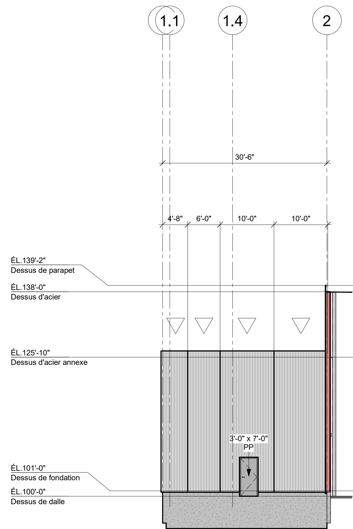
ÉLÉVATION AXE B' (NORD)
